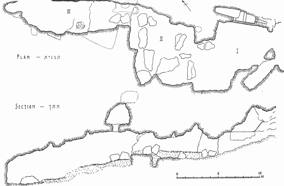
ציור 1 תכנית מערת הברכה
