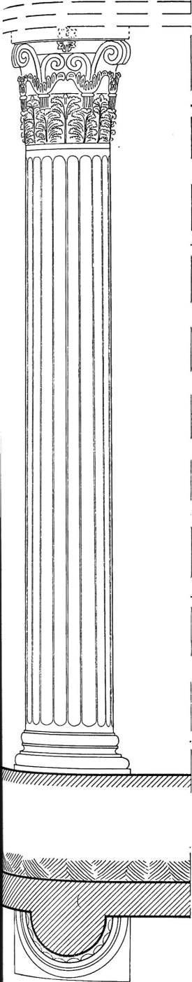
ציור 14. חזית וחתך של עמוד א' דבוק בקיר
