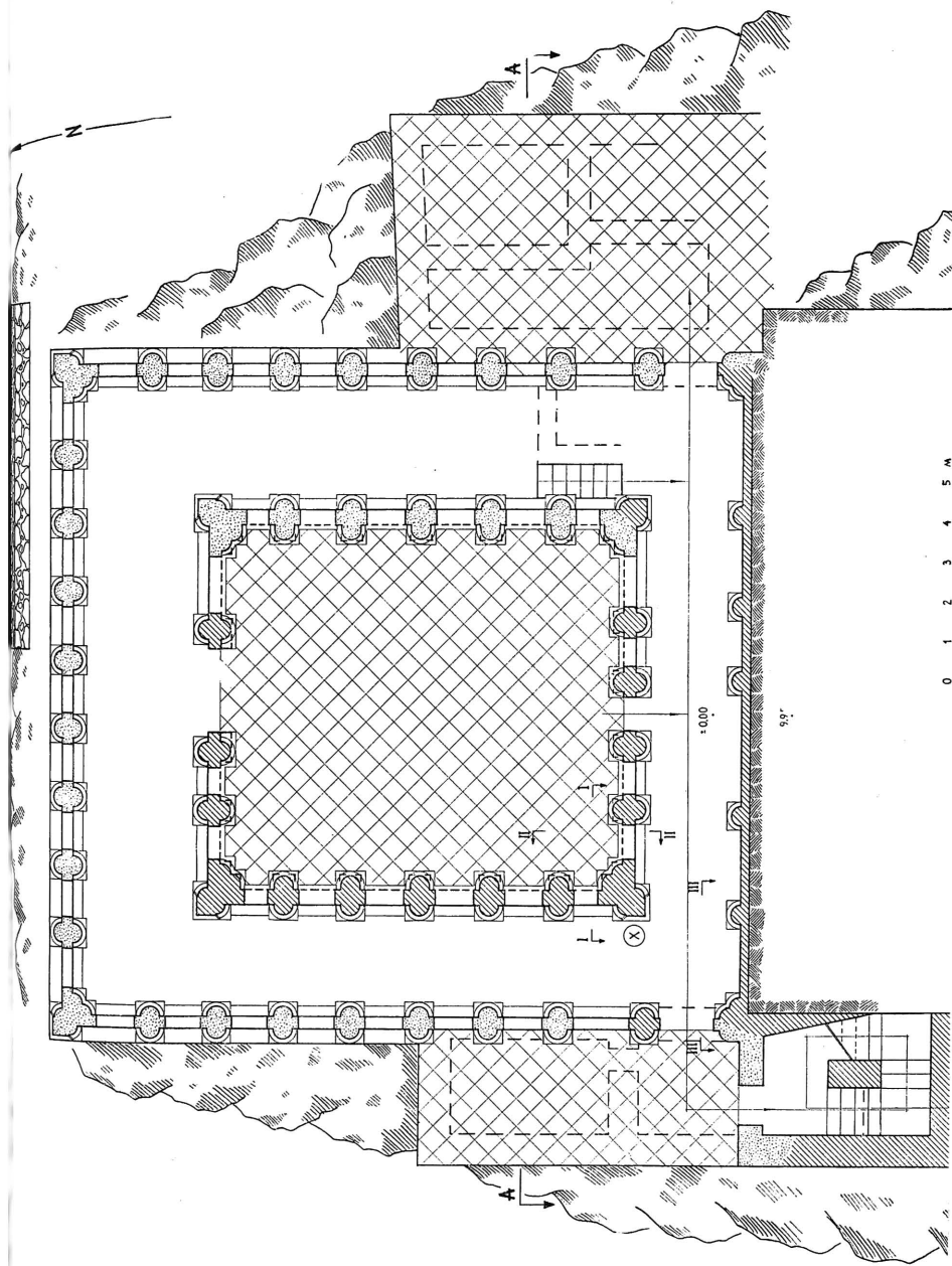
ציור 13. המדרגה התחתונה: תכנית בניין העמודים
