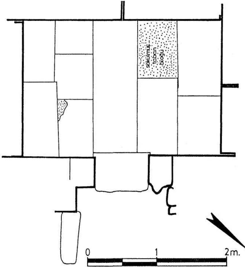
Fig. 1: 1 No.'lu Mezarın Taban Planı
