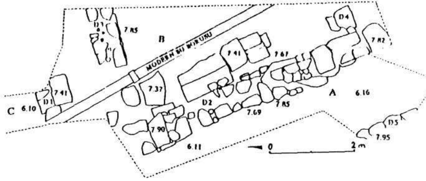
Çiz. 2: II. ve I. Evre Planı
