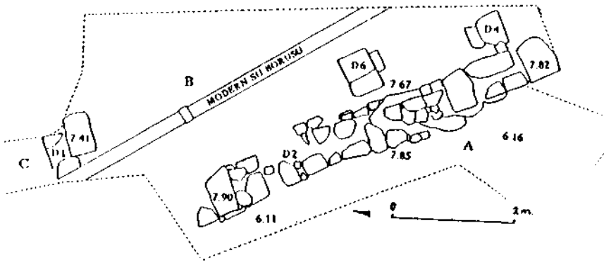
Çiz. 1: III. Evre Planı
